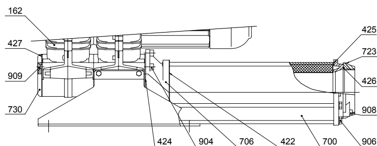
Fig.2 con collettore 90°
