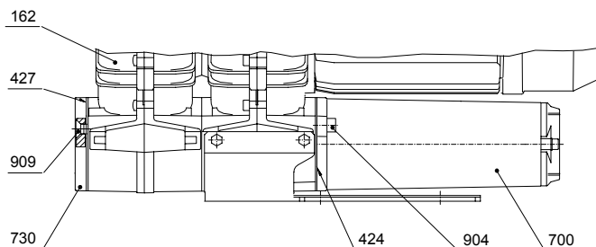
Fig.2 con collettore 90°
