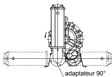
Fig.2 avec adaptateur 90°
