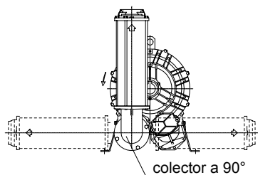
Fig.2 con colector a 90°
