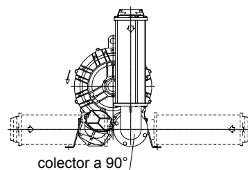
Fig.4 con colector a 90°
