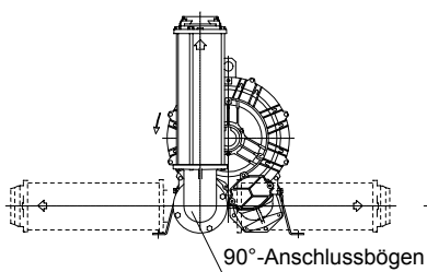
Bild 2 mit 90°-Anschlussbögen
