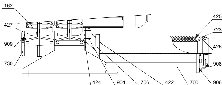
Fig.2 con colector a 90°
