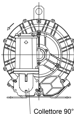
Fig.2 con collettore 90°
