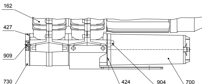
Fig.2 avec adaptateur 90°
