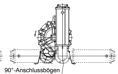
Bild 4 mit 90°-Anschlussbögen
