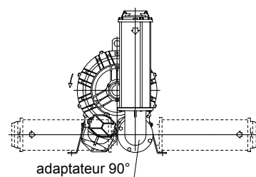
Fig.4 avec adaptateur 90°
