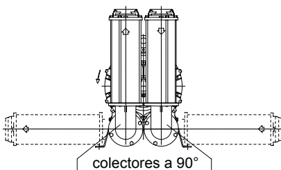
Fig.3 con 2 colectores a 90°
