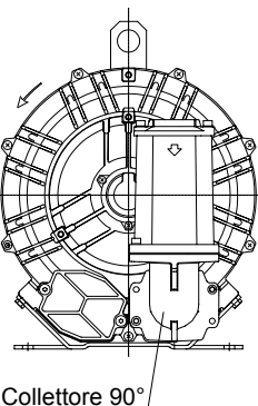
Fig.4 con collettore 90°
