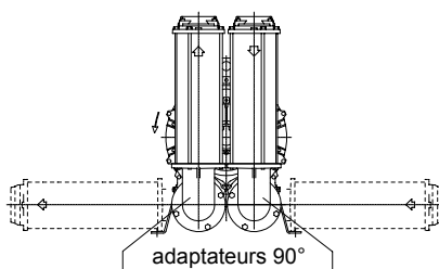
Fig.3 avec 2 adaptateurs 90°
