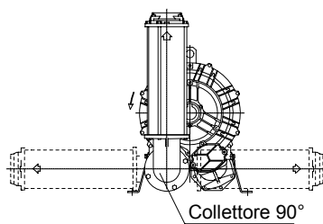
Fig.2 con collettore 90°
