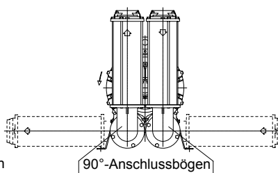
Bild 3 mit zwei 90°-Anschlussbögen
