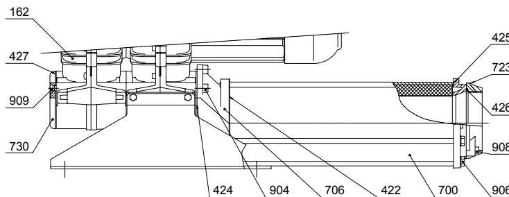
Bild 2 mit 90°-Anschlussbögen
